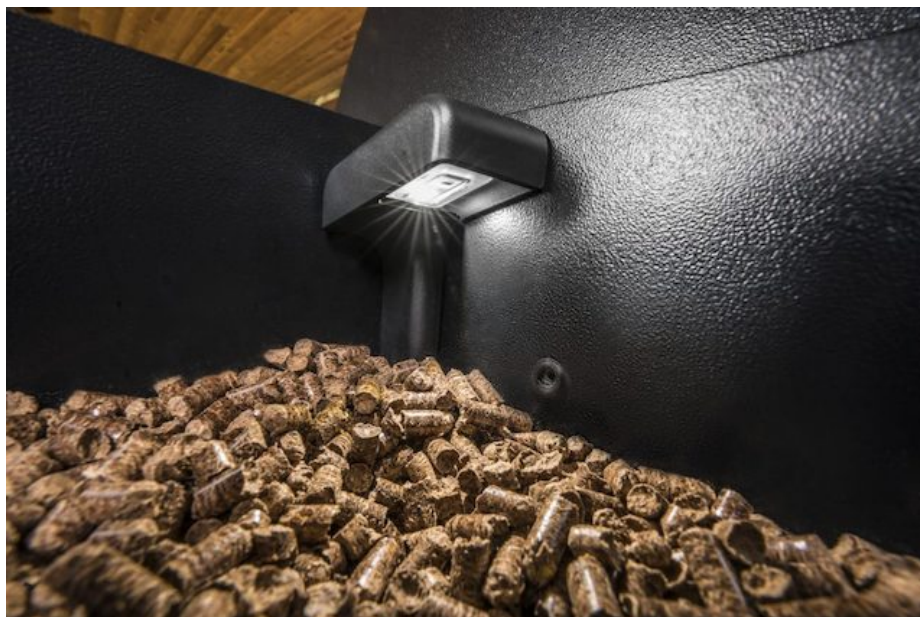
Traeger Pelletsensor til eftermontering
